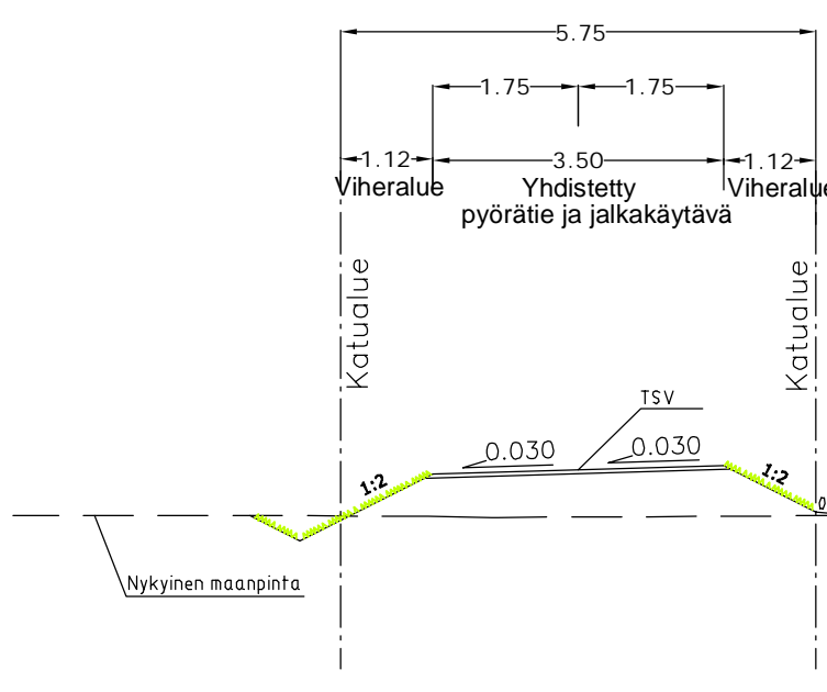
pl 60 Tyypipoikkileikkaus 1:100
