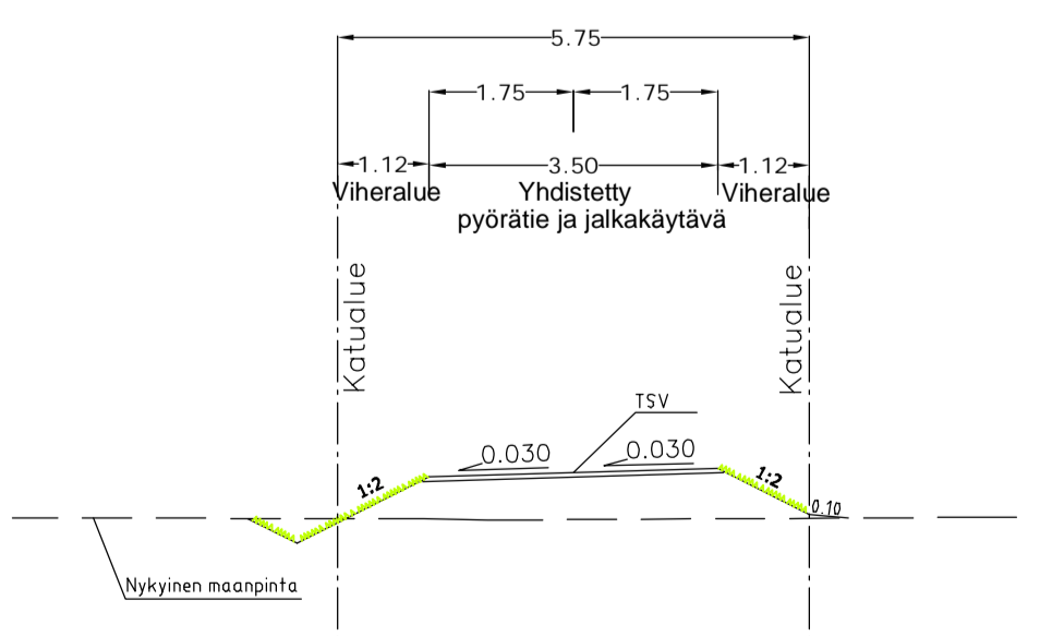
pl 60 Tyypipoikkileikkaus 1:100
